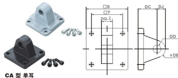
CA 型单耳
